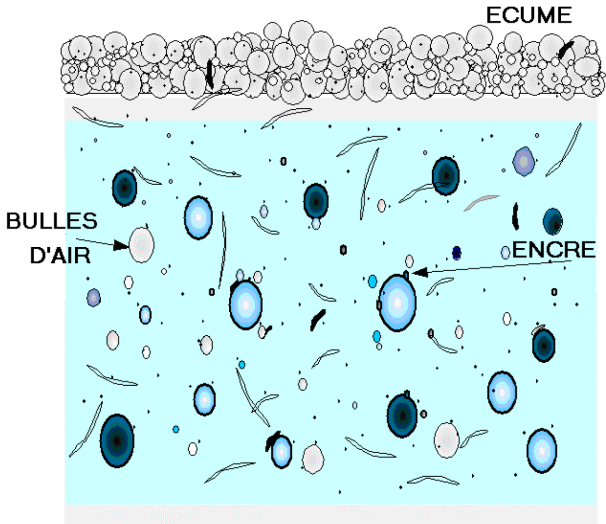
Figure 4: Principe de désencrage par flottation
